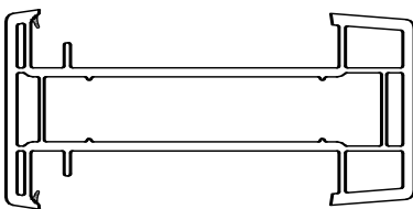
H-Kopplung incl. Dichtung Verstärkung: Art.-Nr. 208 Befestigungsanker: Art.-Nr. AR 152, AL 152, AI 152 Art.-Nr. 352
