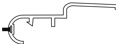
Rolladenkastentraverse mit Dichtung für 10 mm Aufnahme Art.-Nr. 164
