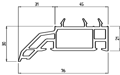
Fensterbank 76 mm Verstärkung: Art.-Nr. 606 Art.-Nr. FB 31
