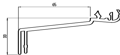
Fensterbankanschluss, 52/65 mm Ausladung Art.-Nr. FB 65
