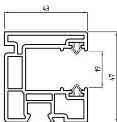
Rolladenführungsschiene mit Dichtung Art.-Nr. 1085
