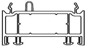
Verbreiterung 30 mm incl. Dichtung Verstärkung: Art.-Nr. 602 Art.-Nr. 360
