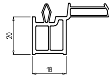
Universalanschluss 20 mm Art.-Nr. 345
