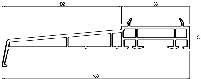
Fensterbank 160 mm Art.-Nr. FB 102
