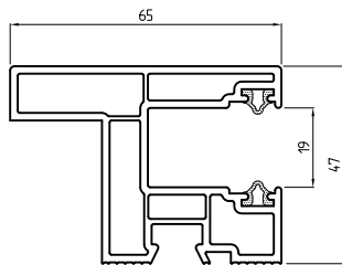
Rolladenführungsschiene mit Dichtung Art.-Nr. 5666
