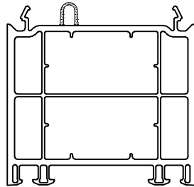
Verbreiterung 60 mm incl. Dichtung Verstärkung: Art.-Nr. 604 Art.-Nr. 362
