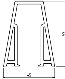
Lisene Verstärkung: Art.-Nr. 205 Art.-Nr. 1114
