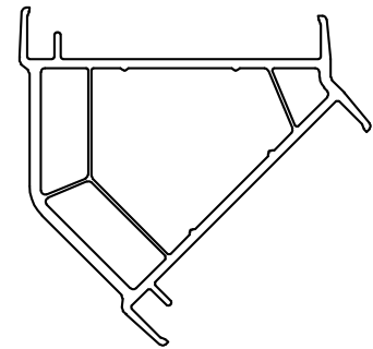
Eckkopplung 135° Verstärkung: Art.-Nr. 656 Art.-Nr. 6356
