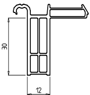
Universalanschluss 30 mm Art.-Nr. 349
