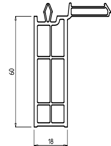
Universalanschluss 60 mm Art.-Nr. 141
