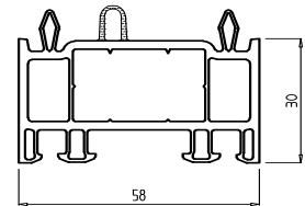
Verbreiterung 30 mm incl. Dichtung Verstärkung: Art.-Nr. 606 Art.-Nr. 144
