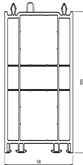
Verbreiterung 120 mm incl. Dichtung Verstärkung: Art.-Nr. S 304020, 219 Art.-Nr. 147
