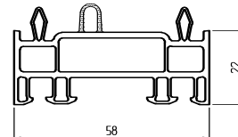
Verbreiterung 22 mm Art.-Nr. 741
