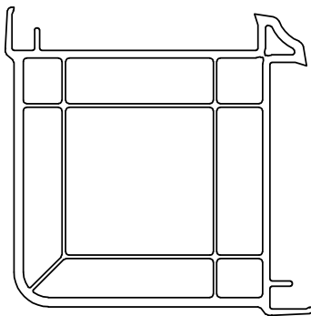
Eckkopplung 90° Verstärkung: Art.-Nr. 655 Art.-Nr. 355
