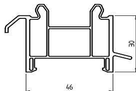
Bankanschluss 30 mm Art.-Nr. 7343
