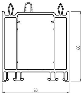
Verbreiterung 60 mm Verstärkung: Art.-Nr. S 304020, 219 Art.-Nr. 546
