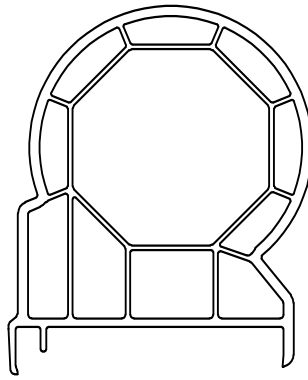
Variable Eckkopplung Verstärkung: Art.-Nr. 640 Art.-Nr. 340
