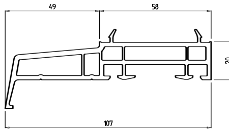
Fensterbank 107 mm Art.-Nr. FB 49
