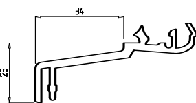
Fensterbankanschluss, 21/34 mm Ausladung Art.-Nr. FB 34
