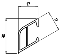
Wetterschenkel 17 x 17 mm Art.-Nr. 174
