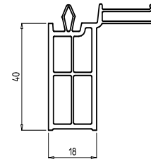
Universalanschluss 40 mm Art.-Nr. 348
