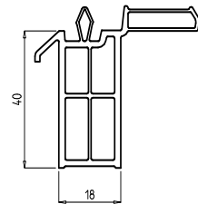
Universalanschluss 40 mm Art.-Nr. 344
