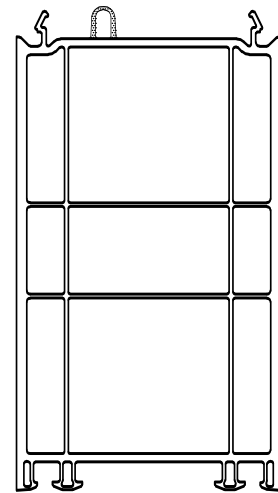
Verbreiterung 120 mm incl. Dichtung Verstärkung: Art.-Nr. 655 Art.-Nr. 363
