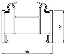
Bankanschluss 30 mm Art.-Nr. 342
