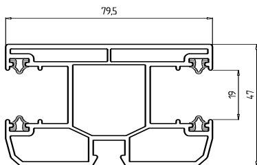
doppelte Rolladen- führungsschiene mit Dichtung Art.-Nr. 4095
