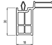
Universalanschluss 30mm Art.-Nr. 346
