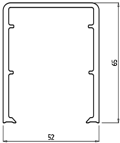
Lisene Verstärkung: Art.-Nr. 614, S 604025 Art.-Nr. 154
