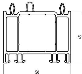
Verbreiterung 45 mm incl. Dichtung Verstärkung: Art.-Nr. 634 Art.-Nr. 545
