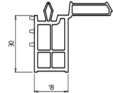
Universalanschluss 30 mm Art.-Nr. 346F
